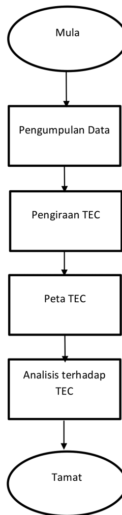
RAJAH 3. Carta alir yang menunjukkan aliran pemprosesan data untuk menghasilkan TEC dan analisis berkaitan
